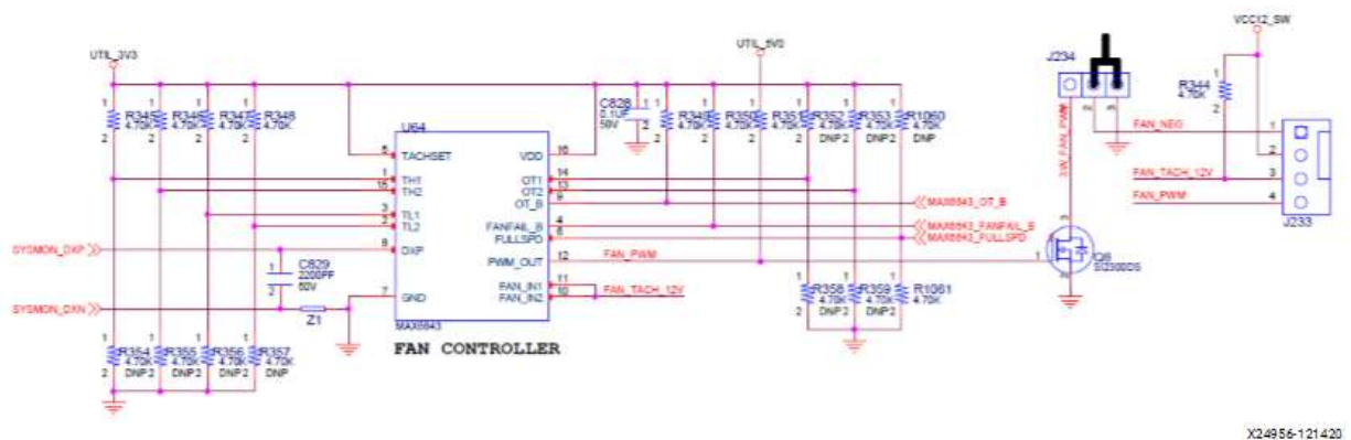
Figure: 12V Fan Header
