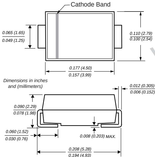
DO-214AC (SMA)
