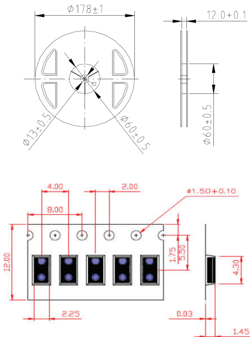
Fig. 16 - Reel Dimensions
