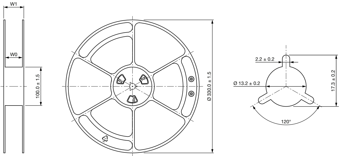
Fig. 17 - Reel Dimensions
