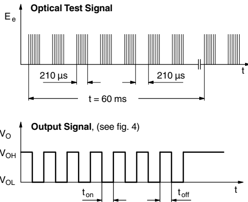
Fig. 3 - Output Function
