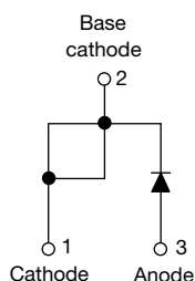
TO-220AC
