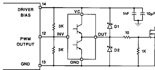
D1, D2: UC3611 Schottky Diode
