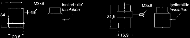
Isolierhülle nur für Variante 250V Insolation only for 250V insert
