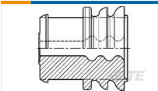
TE Model / Part #963243-1 EINZELDRAHTDICHTUNG
