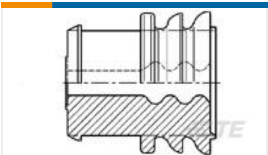
TE Model / Part #963244-1 EINZELDRAHTDICHTUNG
