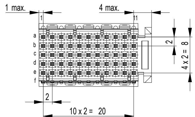
Bestückungsplan / contact layout
