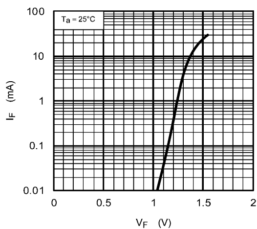
Fig. 12.1.3 I_F - V_F
