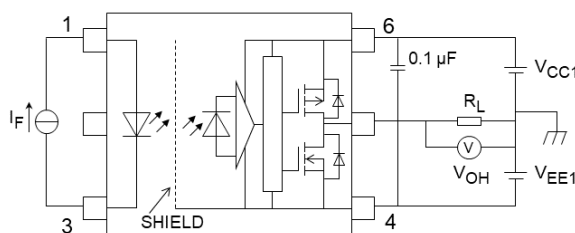
Fig. 13.1.3 V_{OH} Test Circuit
