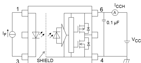
Fig. 13.1.5 I_{CCH} Test Circuit
