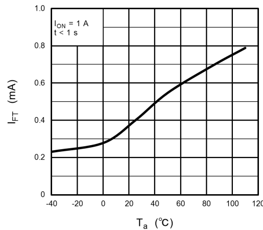
Fig. 13.1.6 I_{FT} - T_a
