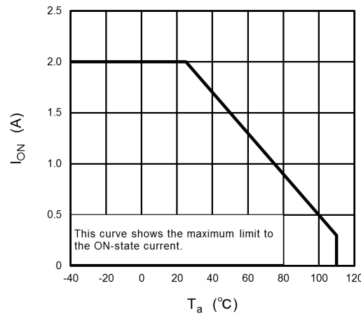
Fig. 13.1.2 I_{ON} - T_a
