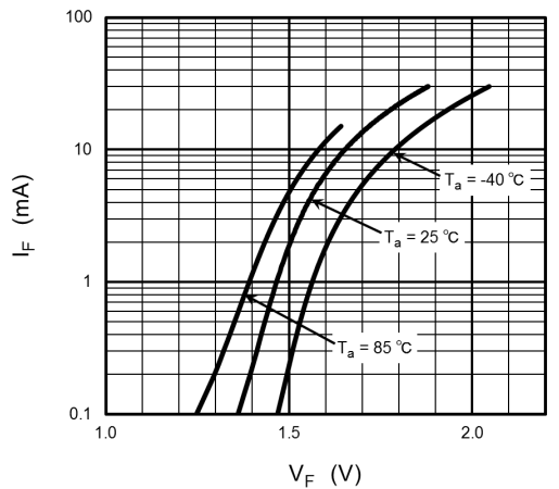
Fig. 13.1.3 I_F - V_F
