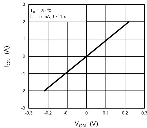
Fig. 13.1.4 I_{ON} - V_{ON}
