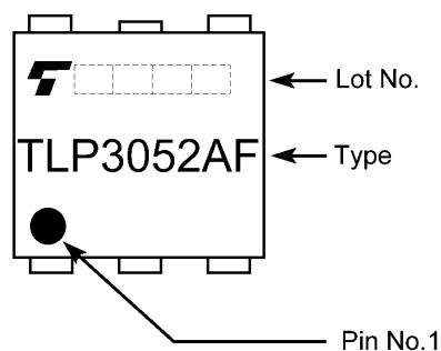
Fig. 15.2 TLP3052AF
