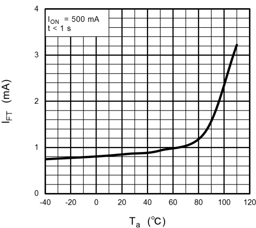
Fig. 12.1.6 I_{FT} - T_a
