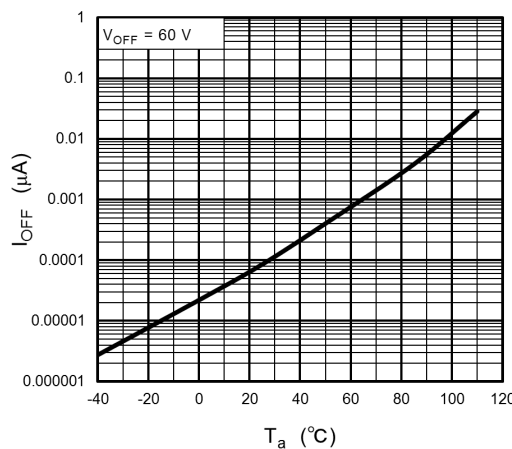
Fig. 12.1.9 I_{OFF} - T_a
