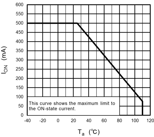
Fig. 12.1.2 I_{ON} - T_a
