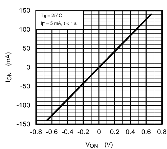
Fig. 12.4 I_{ON} - V_{ON}
