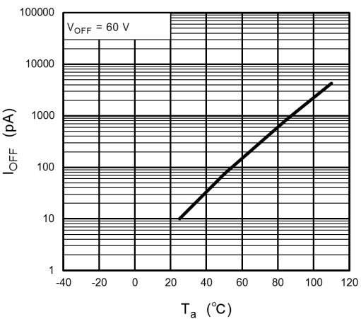
Fig. 12.10 I_{OFF} - T_a
