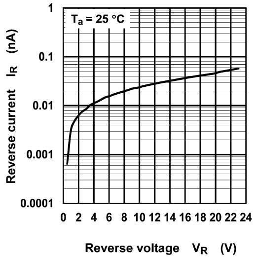
Fig. 8.2 I_R - V_R
