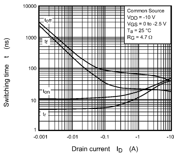
Fig. 7.11 t - I_D
