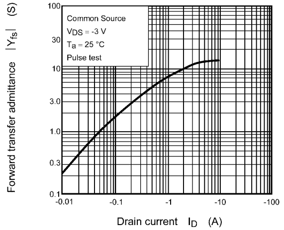
Fig. 7.8 |Y_{fs}| - I_D
