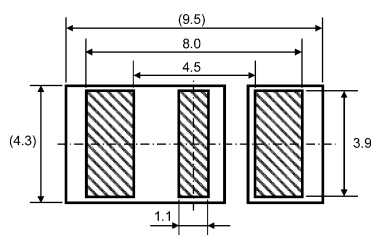
Fig. 10.3.1 (Unit: mm)
