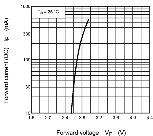
Fig. 8.1 I_F - V_F
