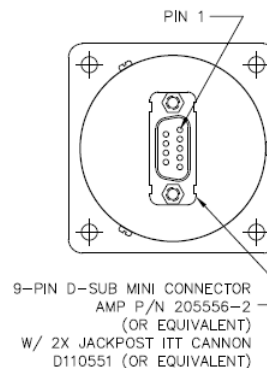
D-Sub
