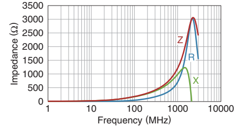
MMZ1005AFZ181V
