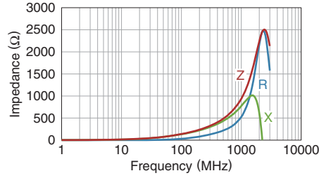
MMZ1005AFZ151V
