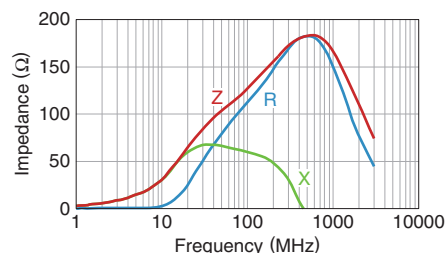
MPZ1608S331ATD25
