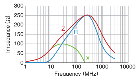
MPZ1608S601ATD25
