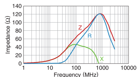
MPZ1608Y600BTD25
