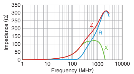
MPZ1005D330ETD25
