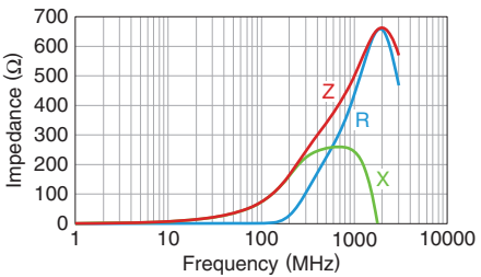
MPZ1005D750ETD25
