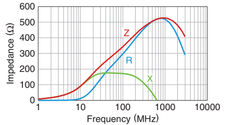
MPZ1005D330ETD25
