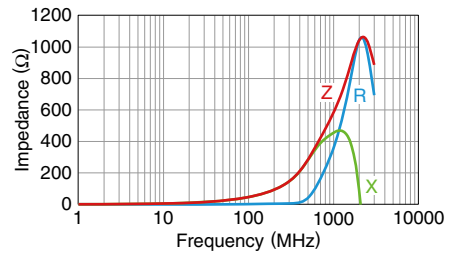
MPZ1005F470ETD25
