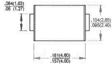
DO-214AC (SMA)
