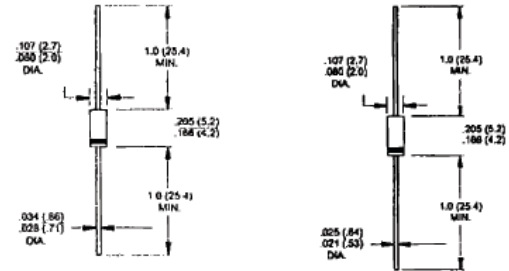
DO-204AL (DO-41)
