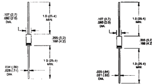
DO-204AL (DO-41)
