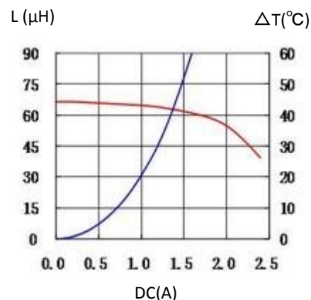
12. CDMPIH10D38NP-680MC
