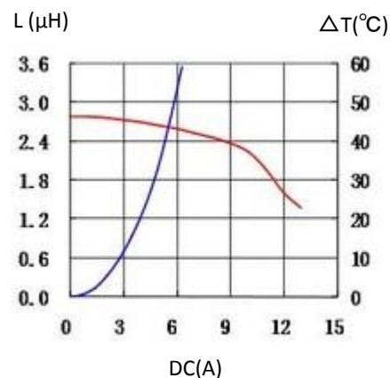
3. CDMPIH10D38NP-2R7PC
