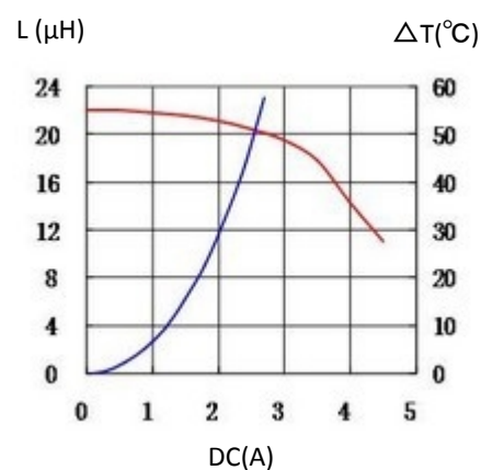
9. CDMPIH10D38NP-220MC
