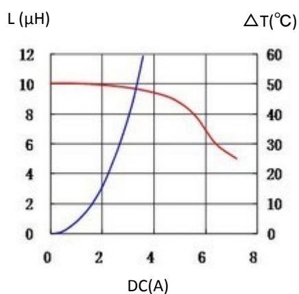
7. CDMPIH10D38NP-100MC
