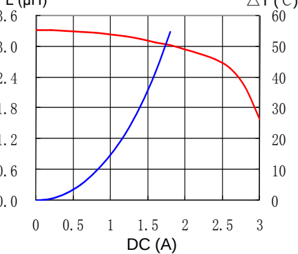
6. CDPH40D18NP-100MC
