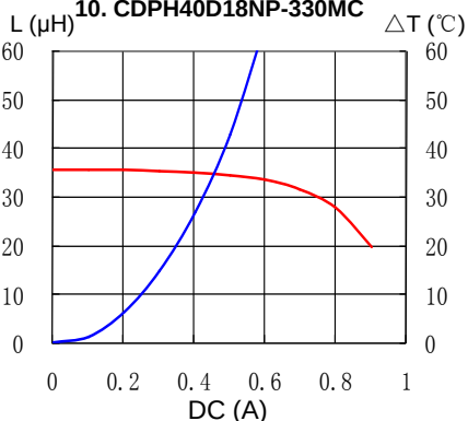
10. CDPH40D18NP-330MC
