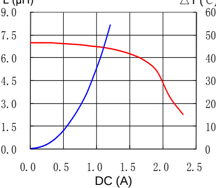
5. CDPH40D18NP-6R8MC
