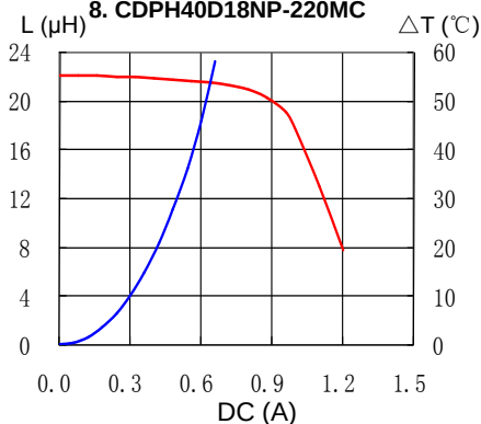
8. CDPH40D18NP-220MC
