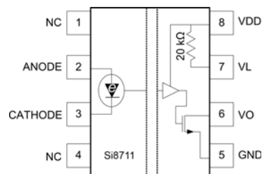
SOIC-8, DIP8
