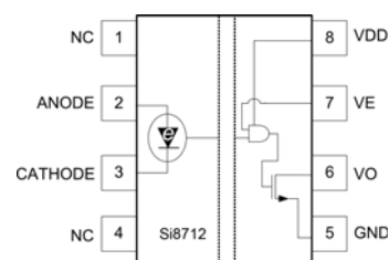
SOIC-8, DIP8
