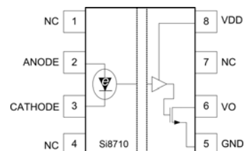
SOIC-8, DIP8
