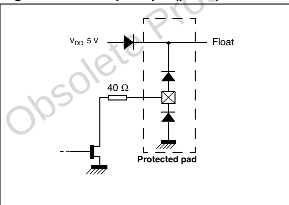
Figure 18. I²C bus (SDA) (Pin 56)
