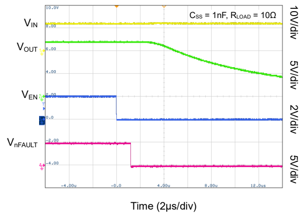
EN Turn-Off Delay: EN↓ to nFAULT↓
