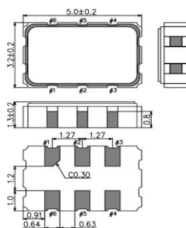
SG5032EEN
