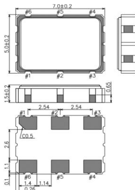
SG7050EEN
