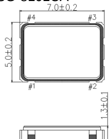
SG-8101CA
