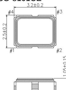
SG-8101CE
