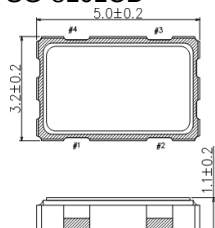
SG-8101CB
