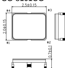
SG-8101CG
