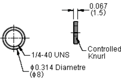
HDW19
