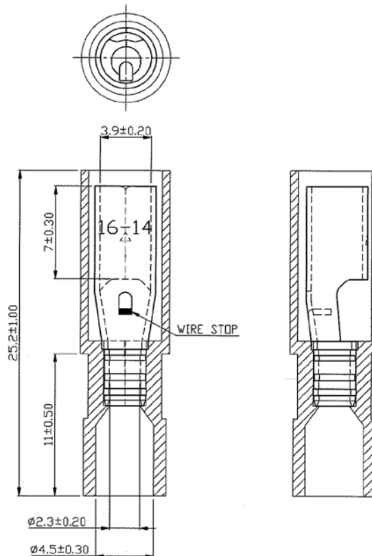
Dimensions : Millimetres
