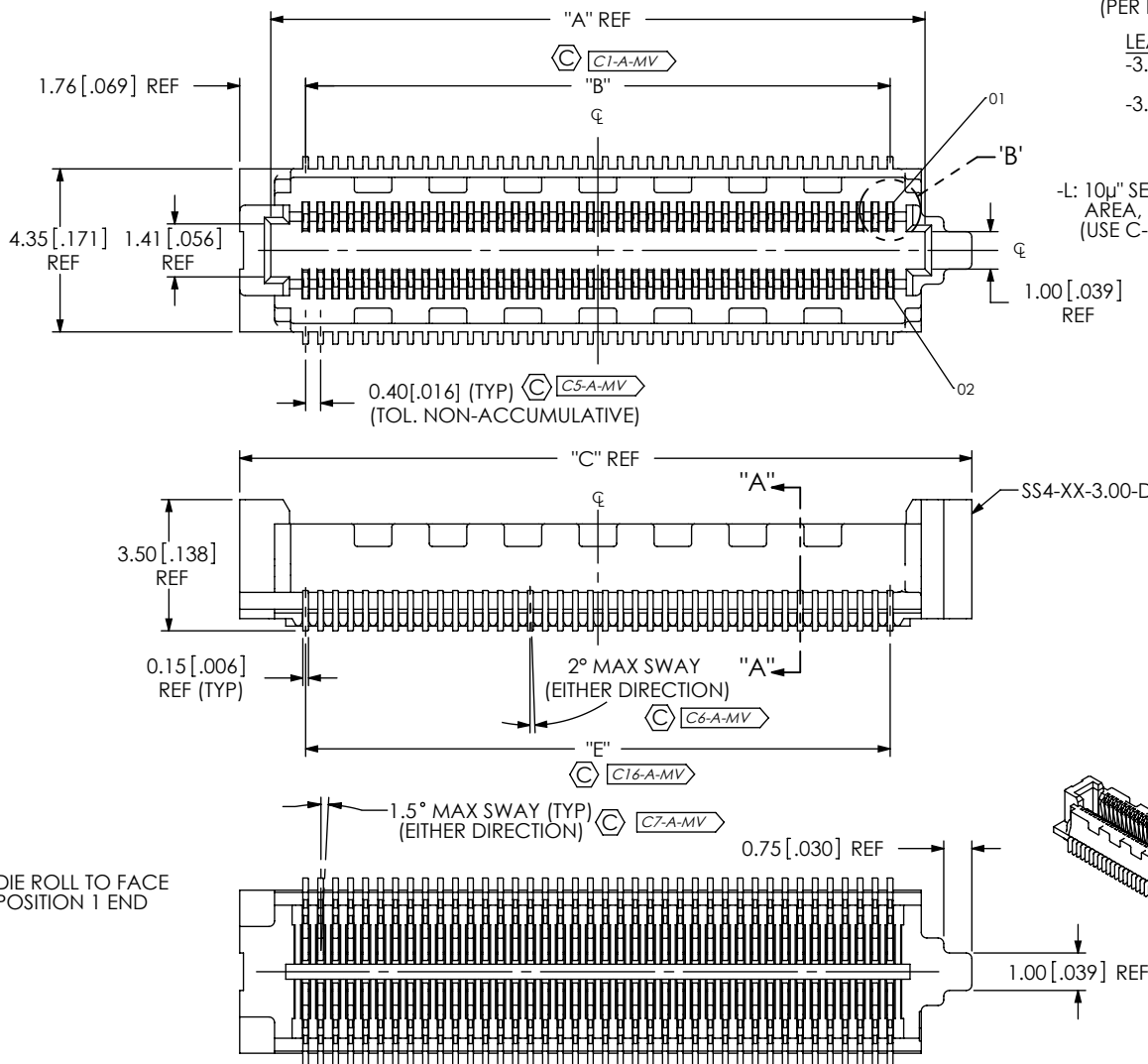
FIG 1 SS4-40-3.00-L-D SHOWN
