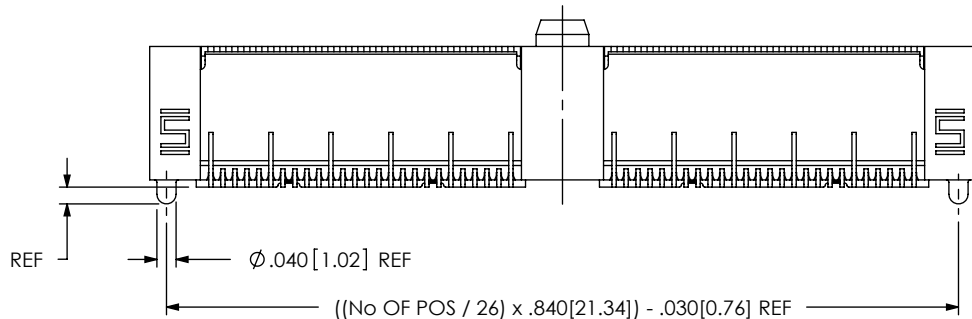
FIG 1 QFSS-052-04.25-X-D-A SHOWN
