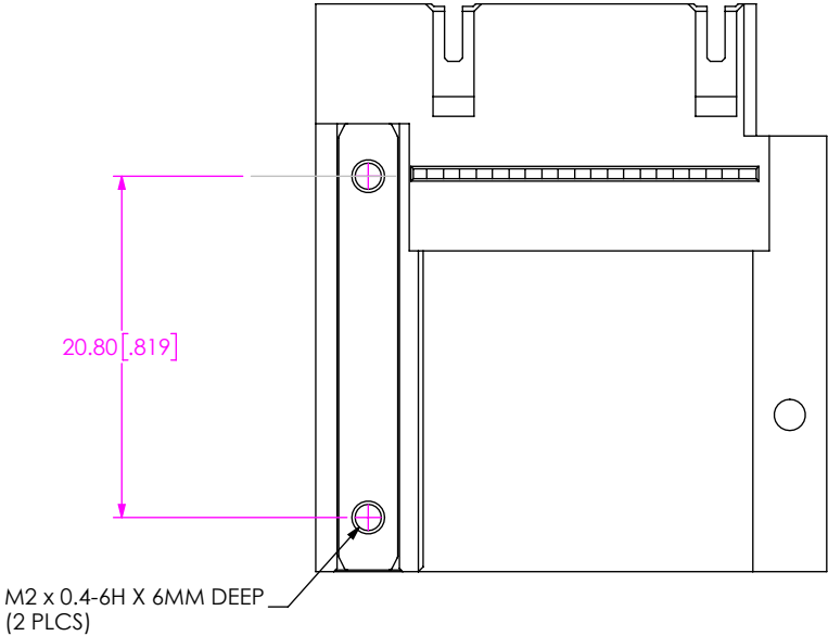
FIG 2 END 2, -R-1-L-G SHOWN
