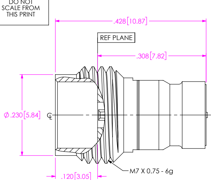
DETAIL 'A' SCALE 10:1
