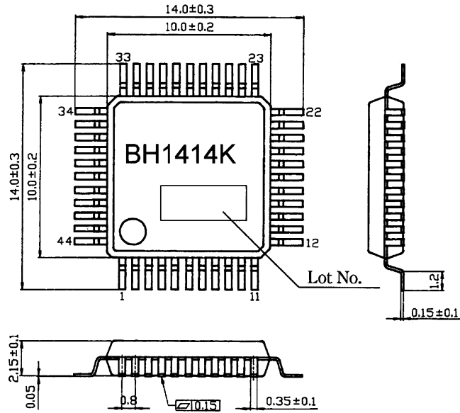
QFP-44(Unit : mm)
