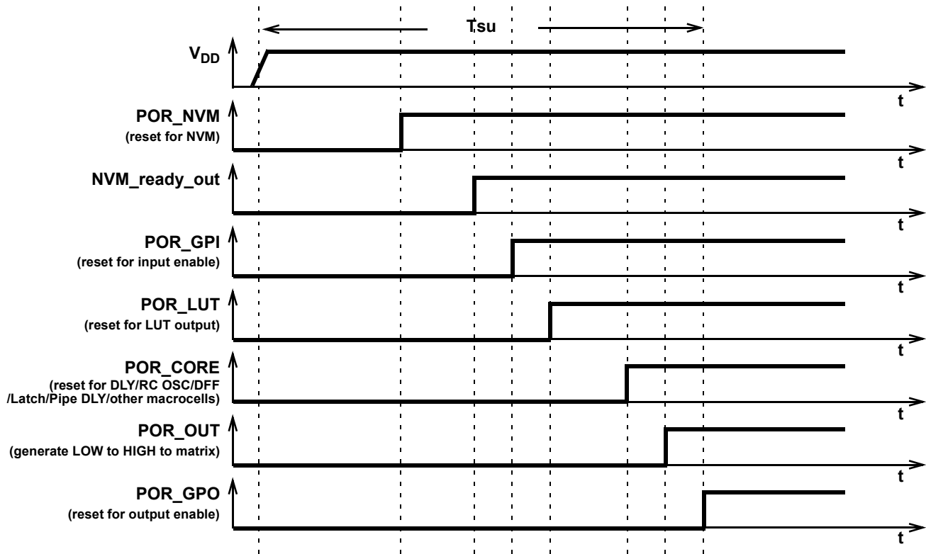
Figure 34. POR Sequence
