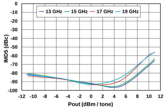
IMD5 vs Pout
