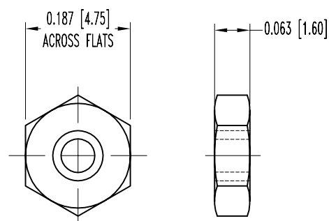
HEX NUT
