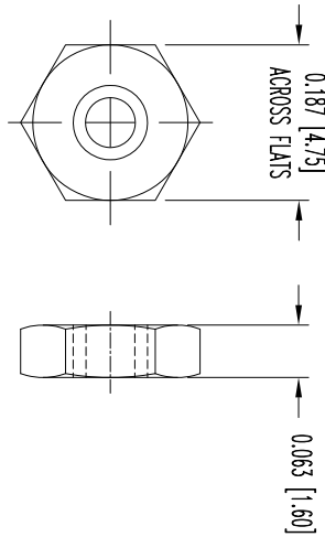
HEX NUT
