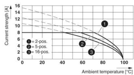
Type: MCVR 1,5/...-ST-3,5 AU with MCV 1,5/...-G-3,5 AU
