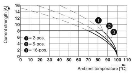
Type: MC 1,5/...-ST(F)-3,5 AU with MCV 1,5/...-G(F)-3,5 AU
