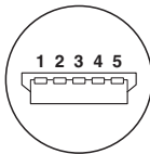
Pin assignment plug USB, mini B
