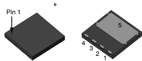
PQFN4 8X8, 2P (Power88) CASE 483AP
