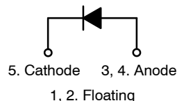
Schottky Diode
