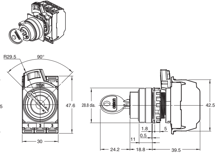
A22NK-2B□-01□A-P
