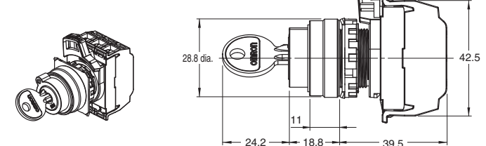
A22NK-2M□-01□A-P
