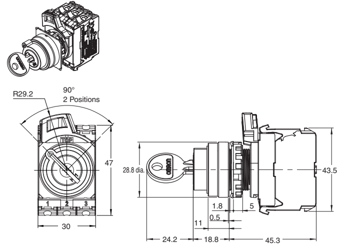
A22NK-2B□-01□A-G
